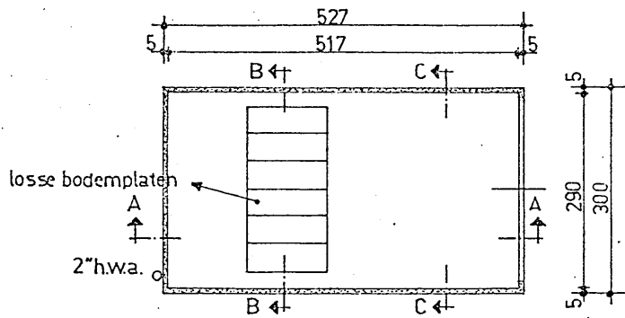
PLATTEGROND
