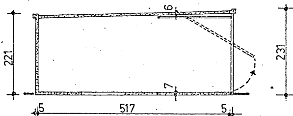
DOORSNEDE A-A
