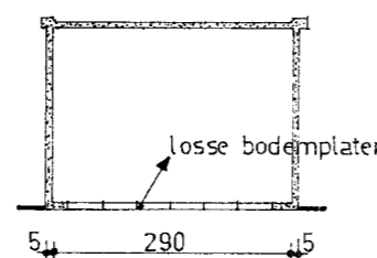
DOORSNEDE B-B
