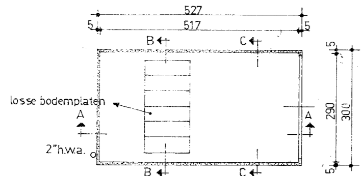
PLATTEGROND
