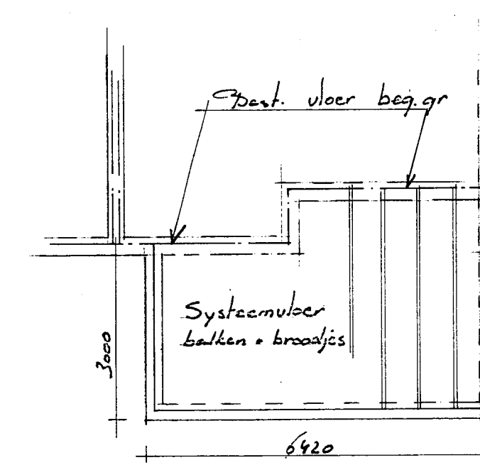
Begane-Grondvloer
