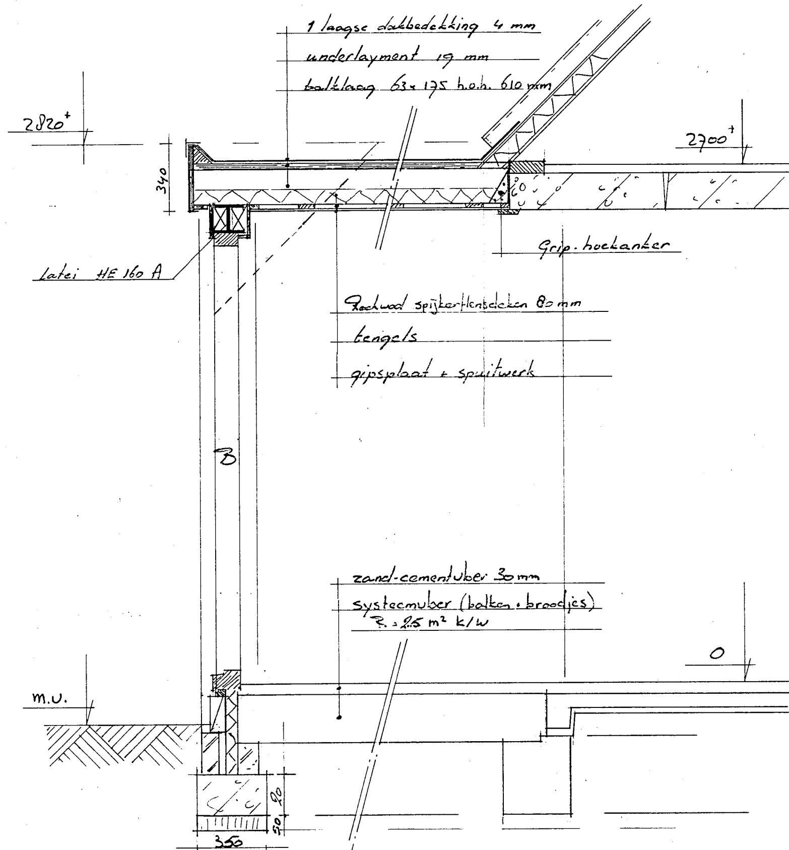
Detail aarbouw
