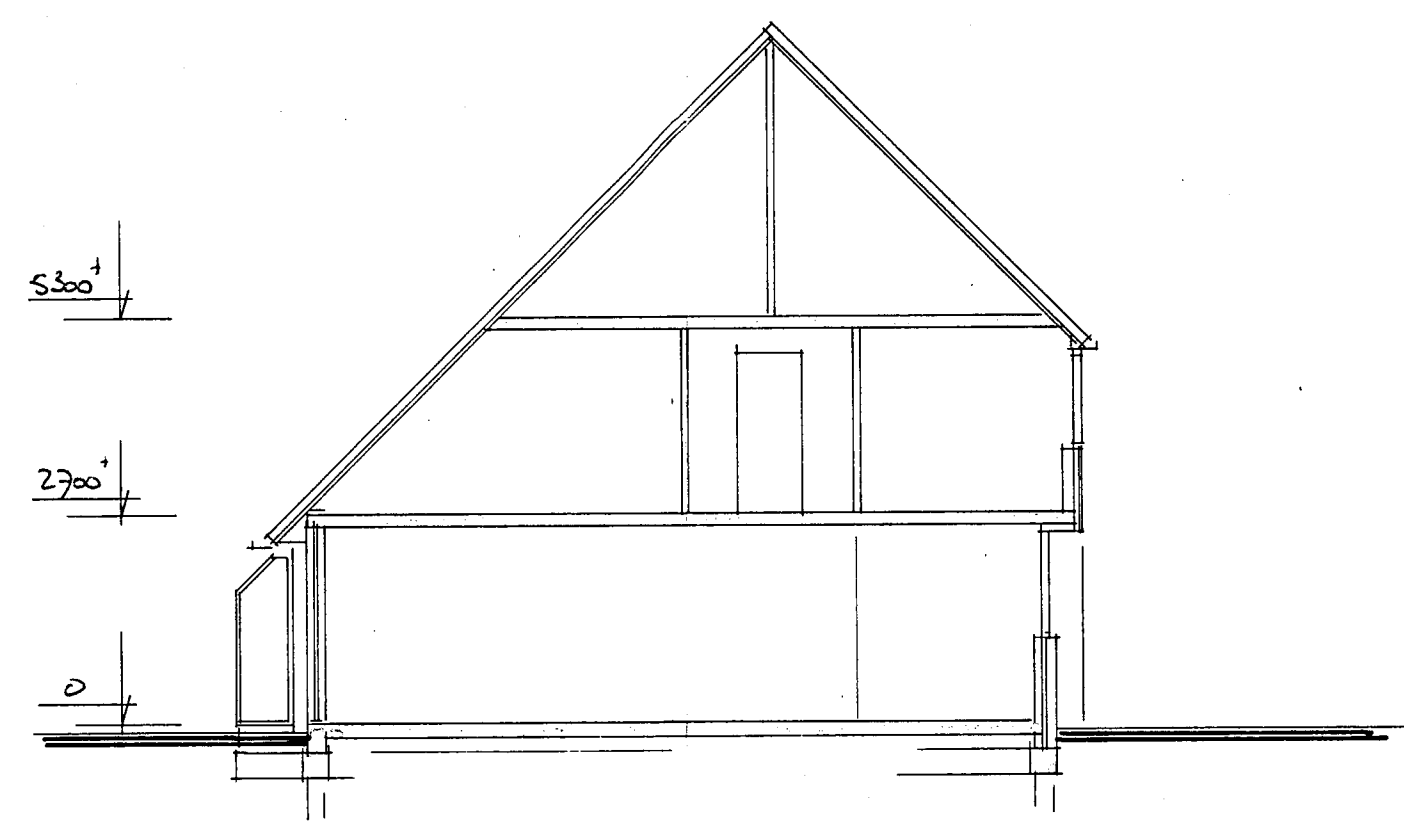
Best. Doorsnede
