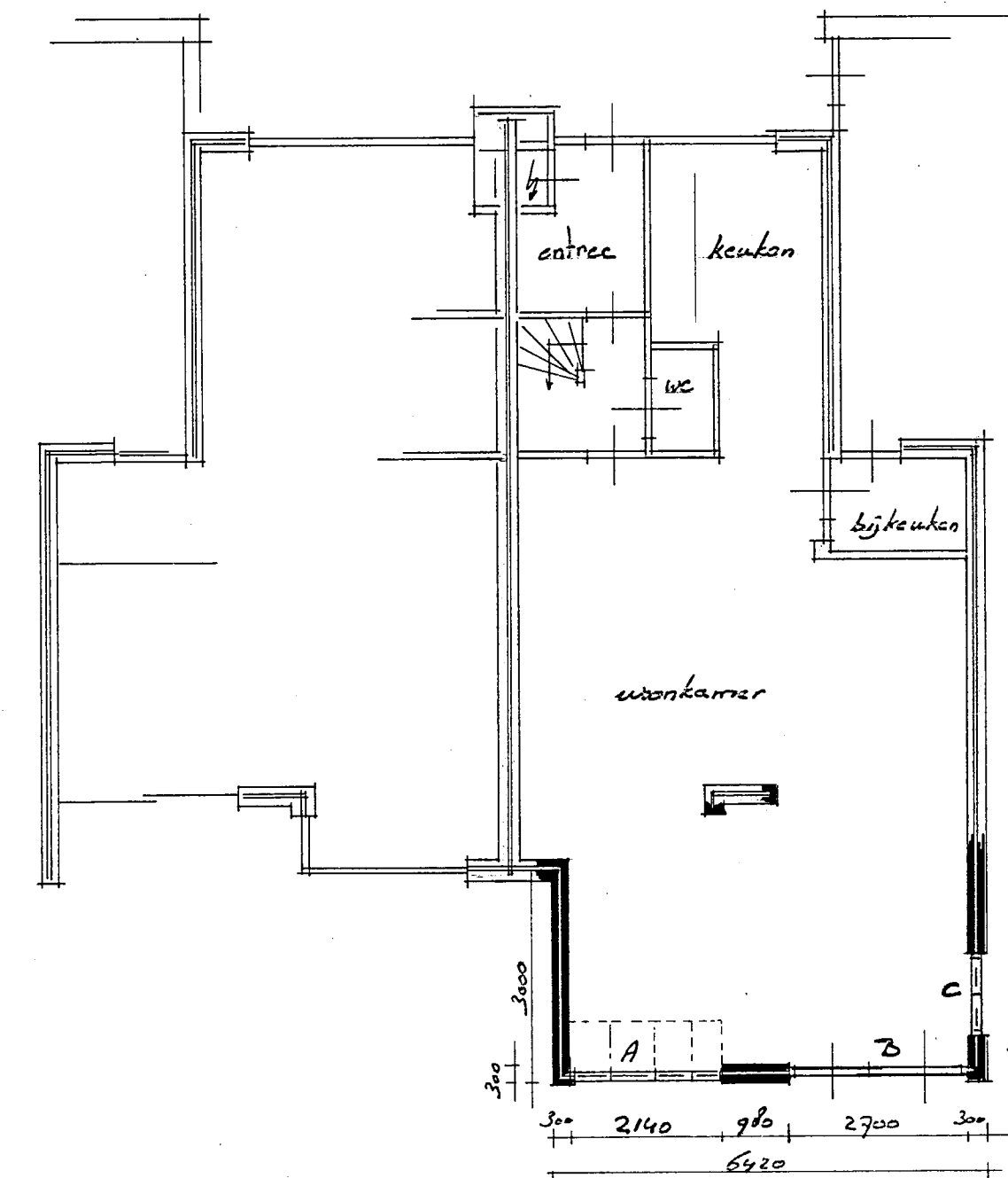
Gen. Begane-Grond
