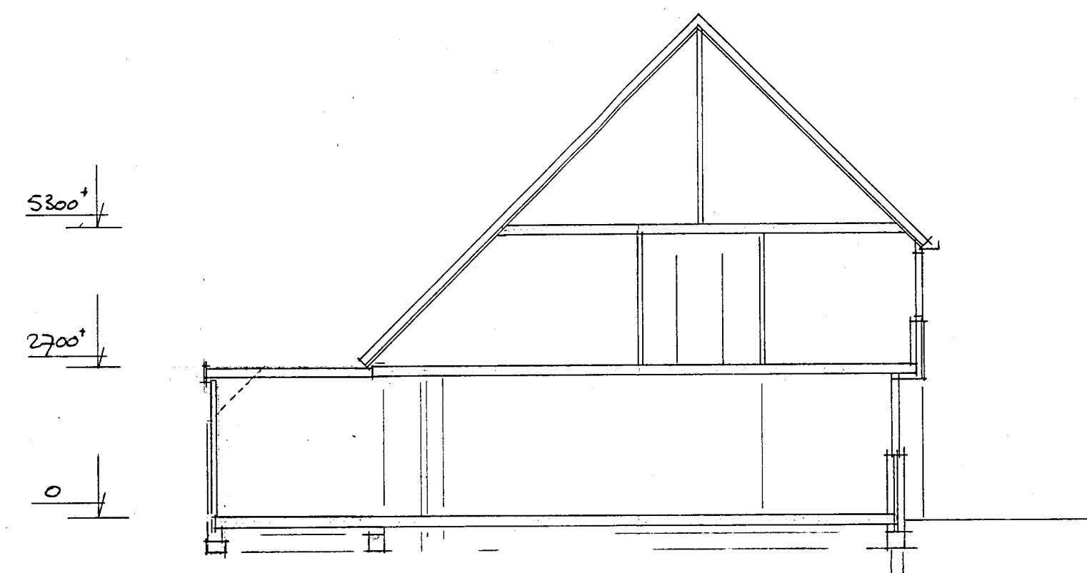
Gen. Doorsnede
