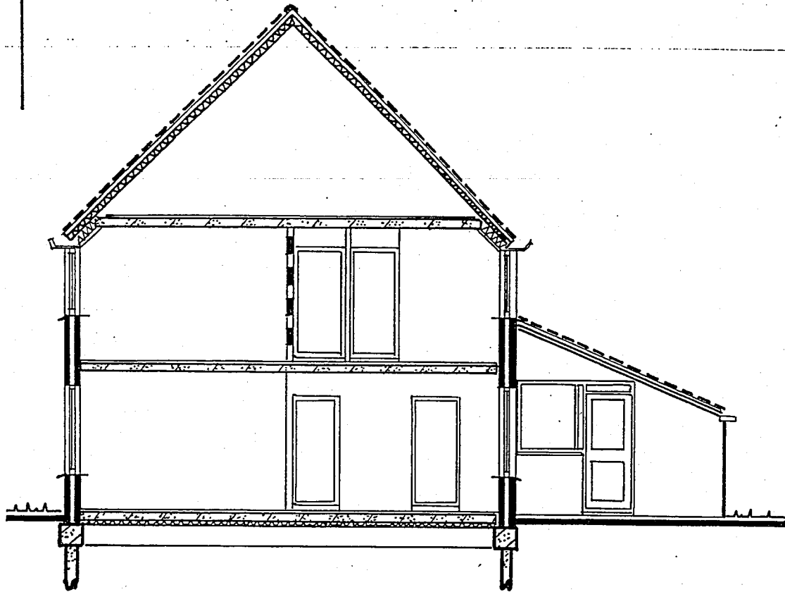
- doorsnede bestaand -
