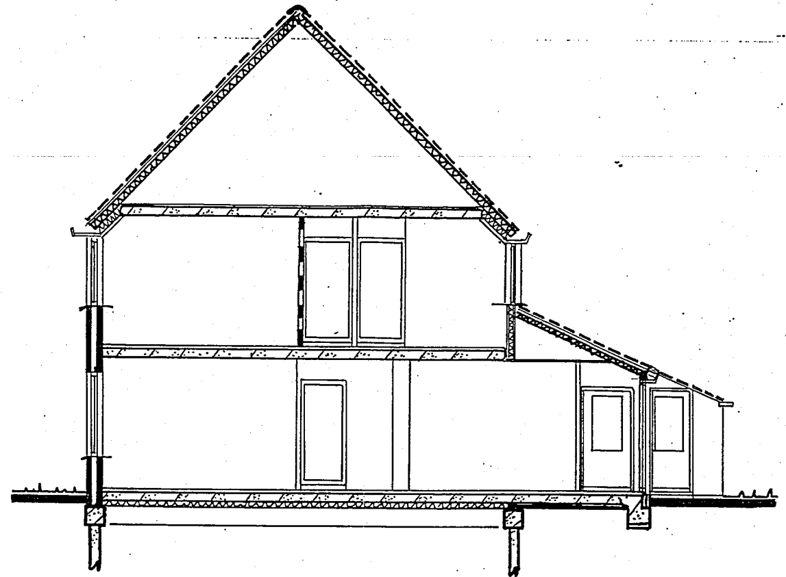
- doorsnede nieuwe situatie -
