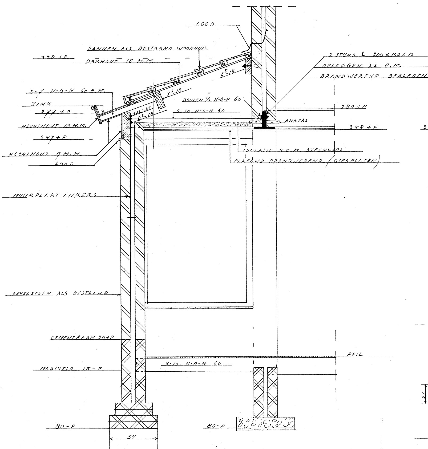
doorsnede - A
