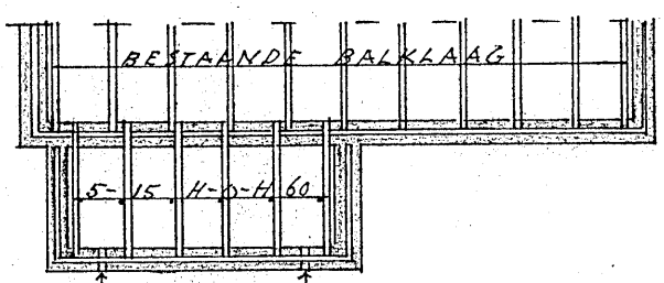
begane grond-balklaag
