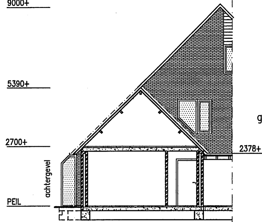
Aanzicht A. -bestaand-
