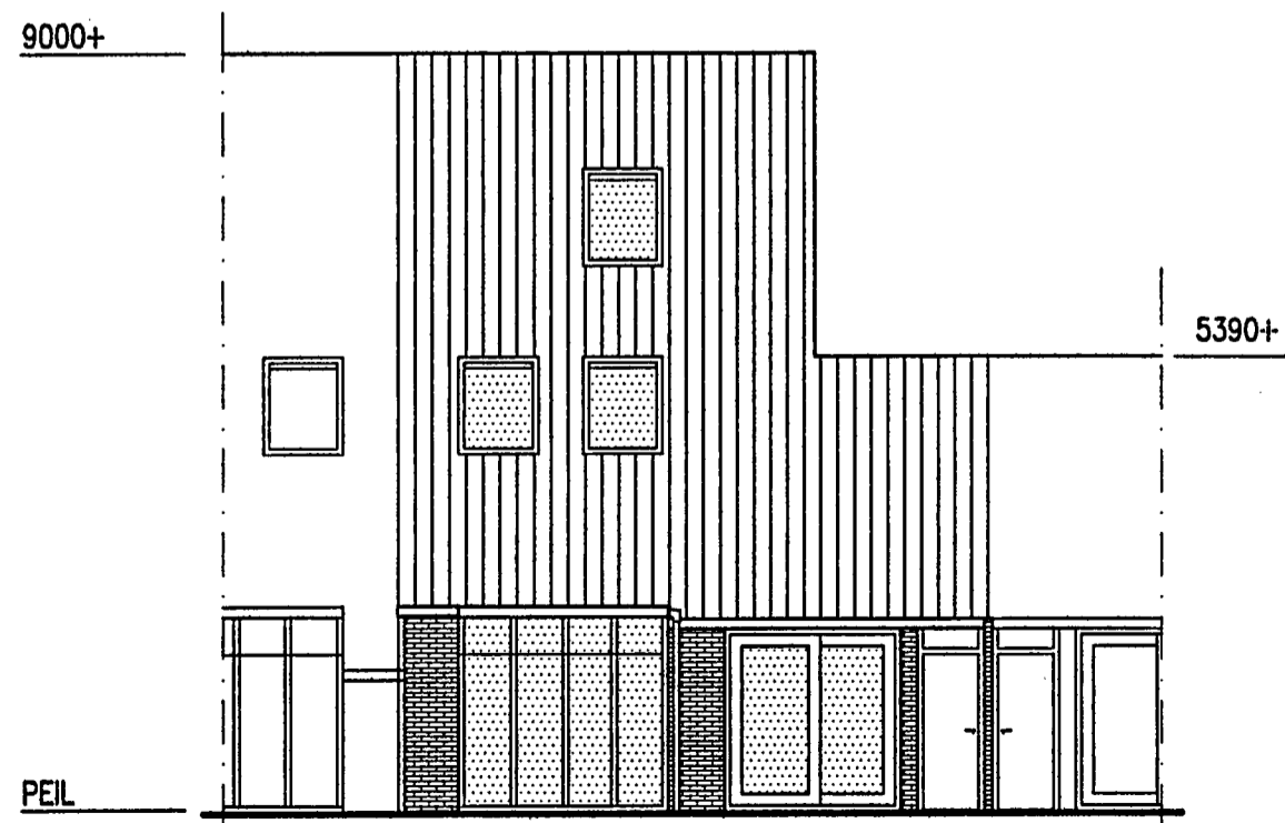
Aanzicht achtergevel -nieuw-
