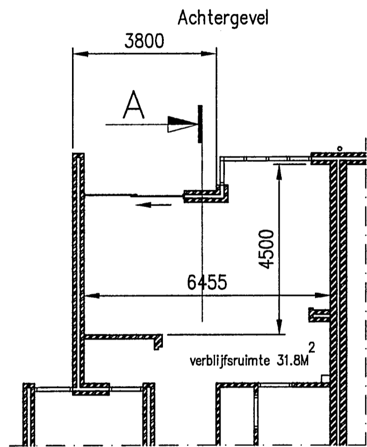
Plattegrond -bestaand-
