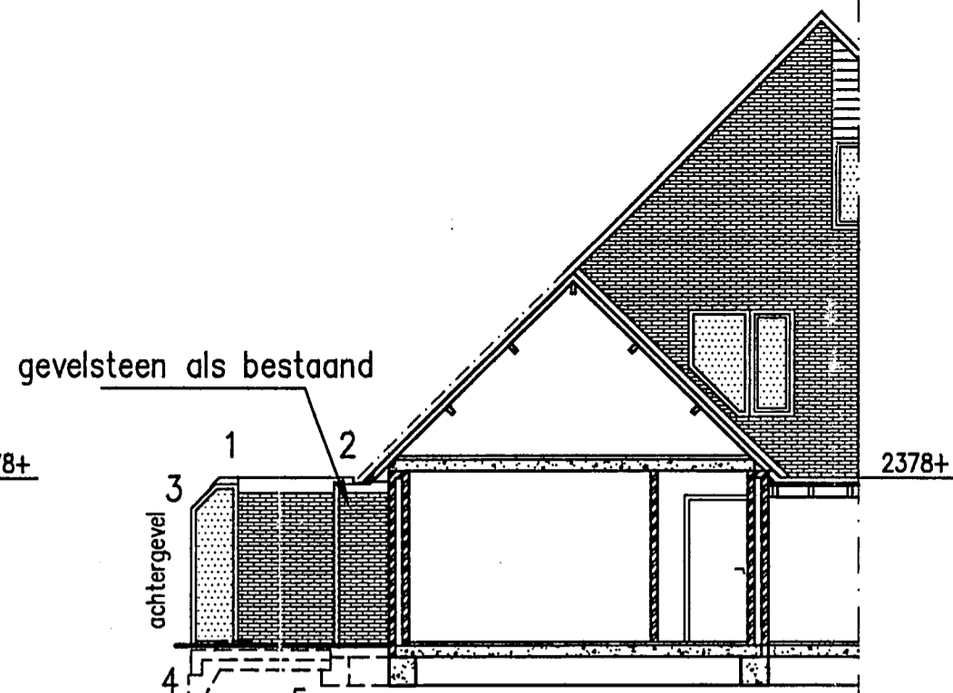
Aanzicht A. -nieuw-
