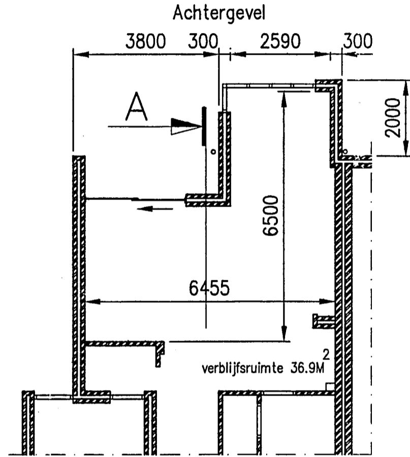
Plattegrond -nieuw-
