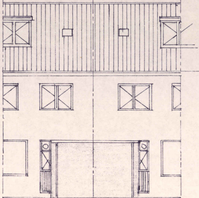
Aanzicht achtergevel met kopwand- bijshuur
