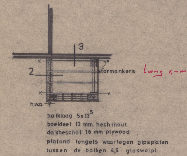
PLATDAK BALKLAAG
