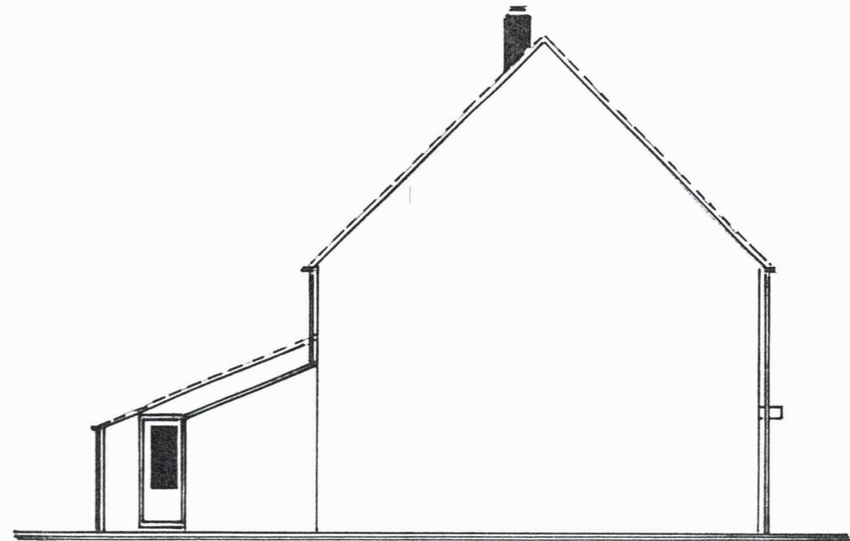
bestaande zijgevel 1:100
