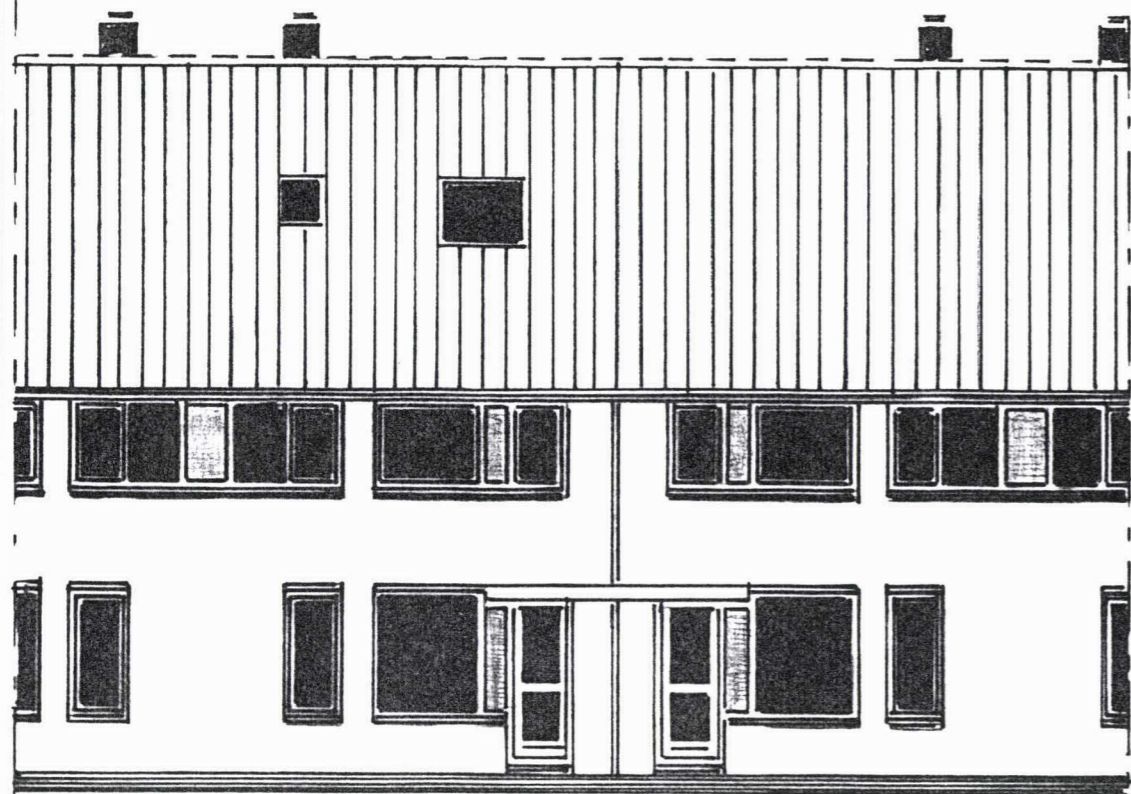
bestaande voorgevel 1:100
