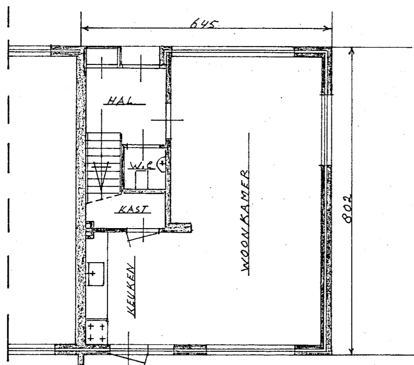
begane grond
