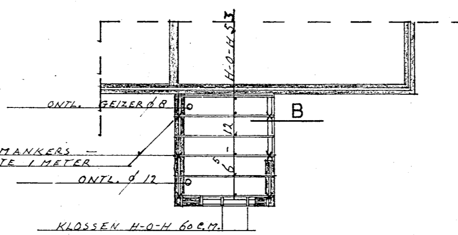
platdak-balklaag
