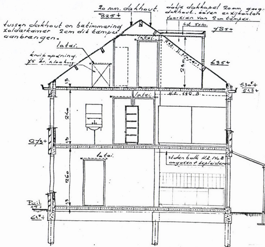
. HOOGTE-DOORSNEDE.
