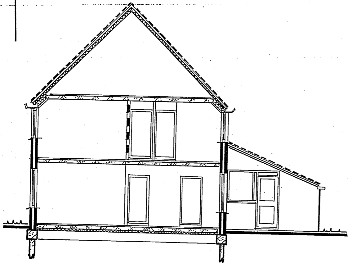
- doorsnede bestaand -
