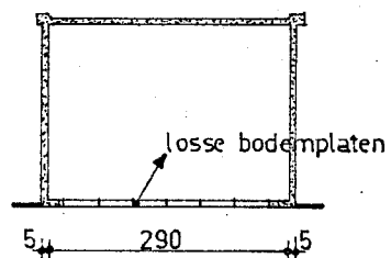
DOORSNEDE B-B
