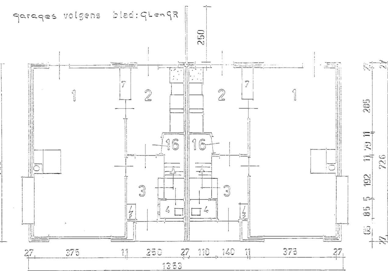
BEGANE GROND
