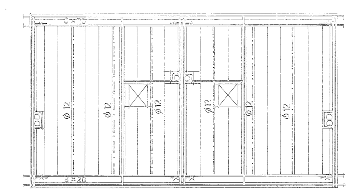
PLAFONDHANGERS 6 x 10 h.o.h. max. 80 cm.
