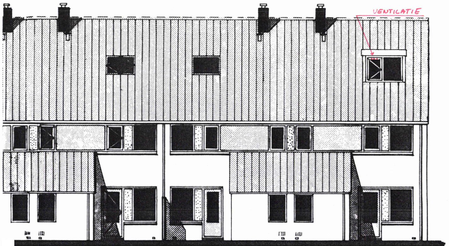
achtergevel
