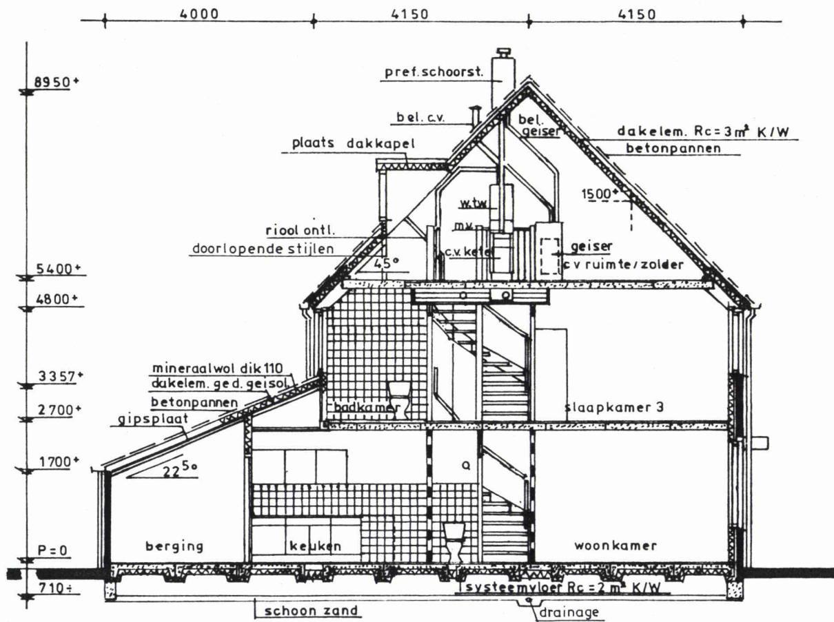
doorsnede
