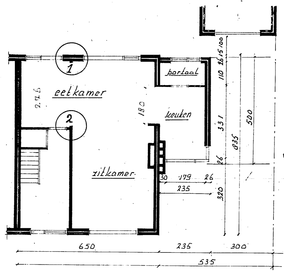
platte grond
