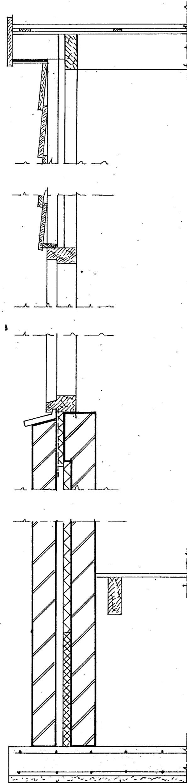
doorsnede A-B
