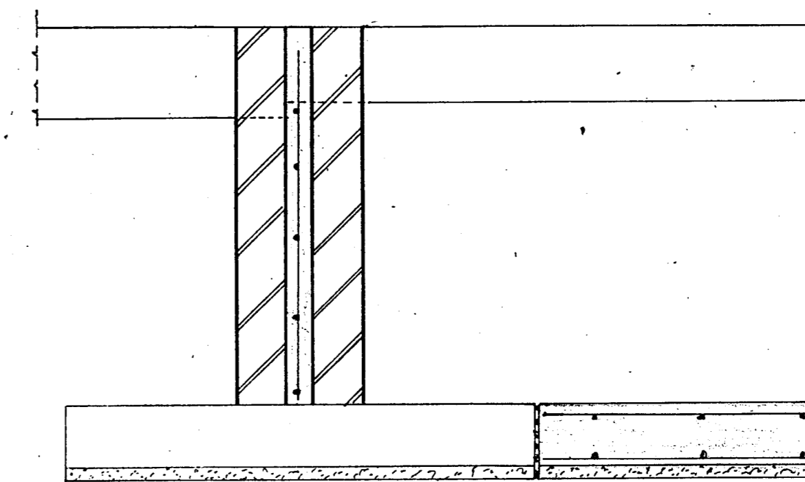
doorsnede C-D
