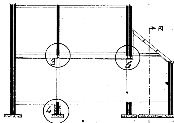
doorsnede
