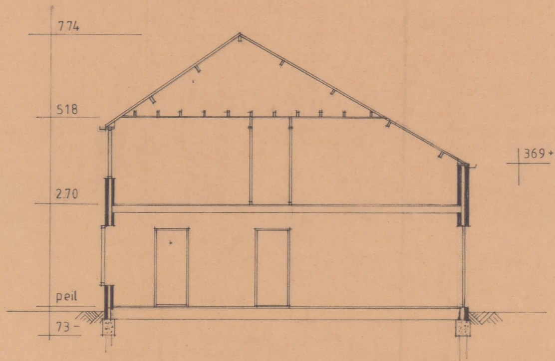
best. doorsnede
