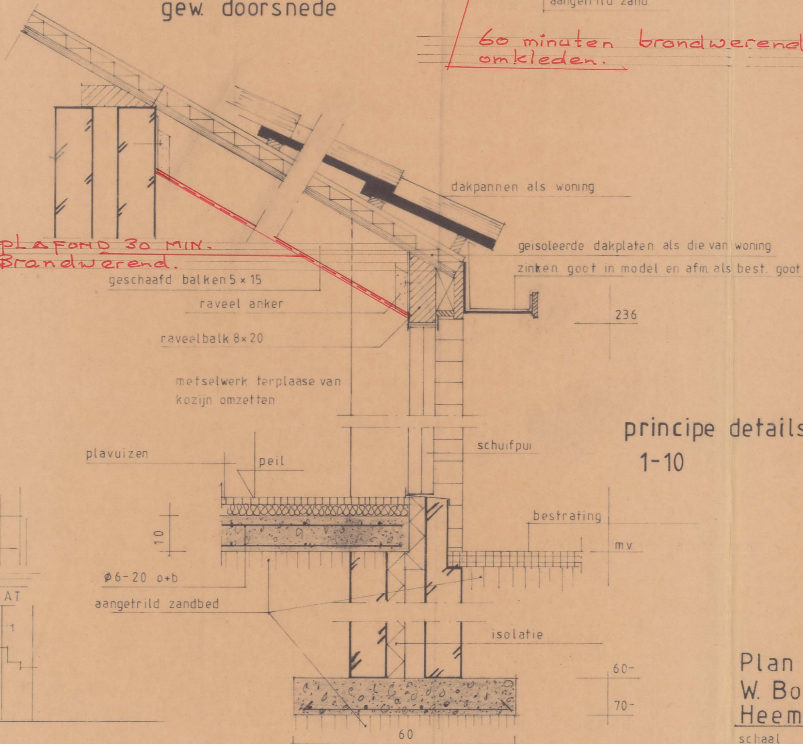
gew. doorsnede
