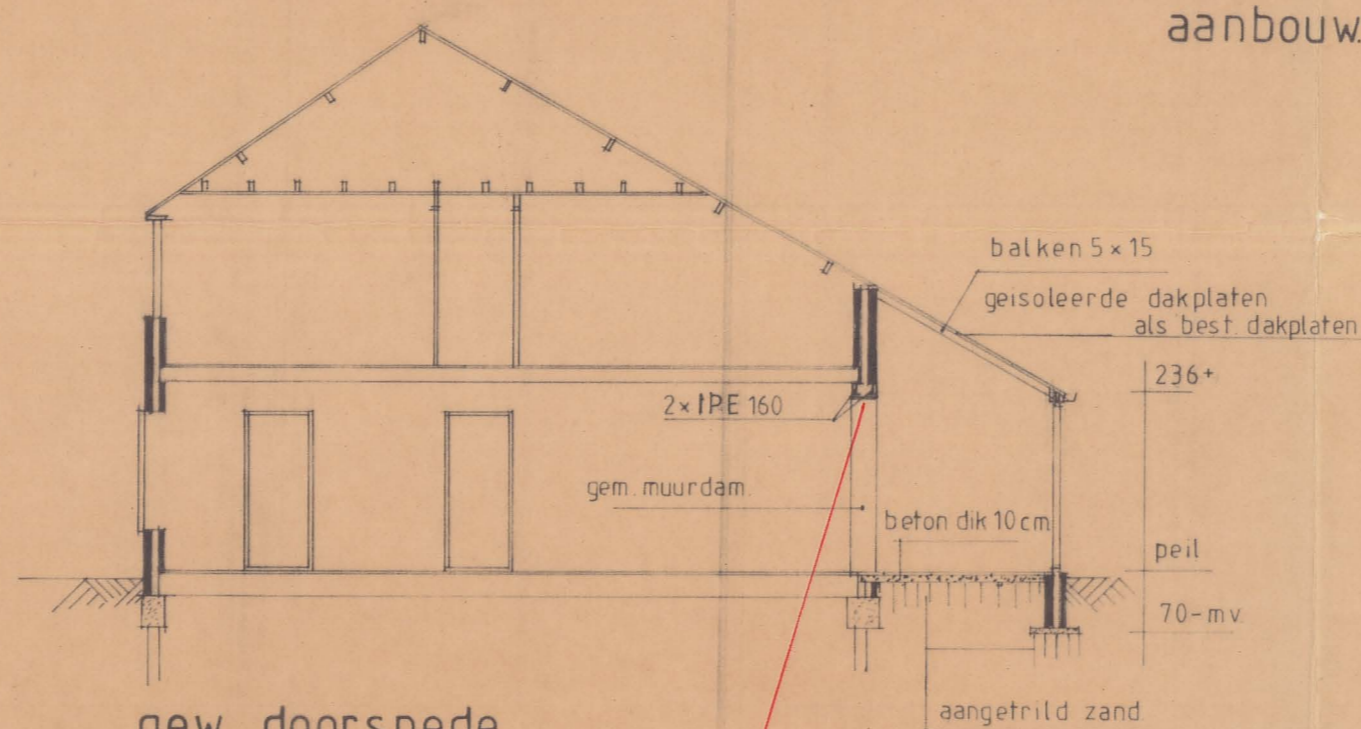
gew. doorsnede
