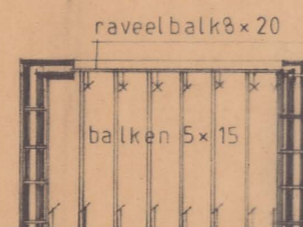
kapplan
