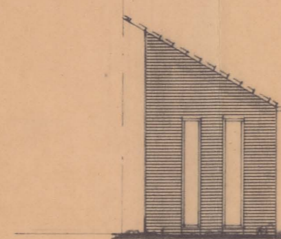
zijaanzicht aanbouw.
