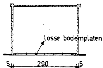
DOORSNEDE B-B
