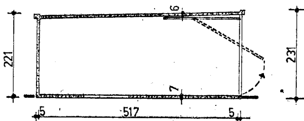
DOORSNEDE A-A
